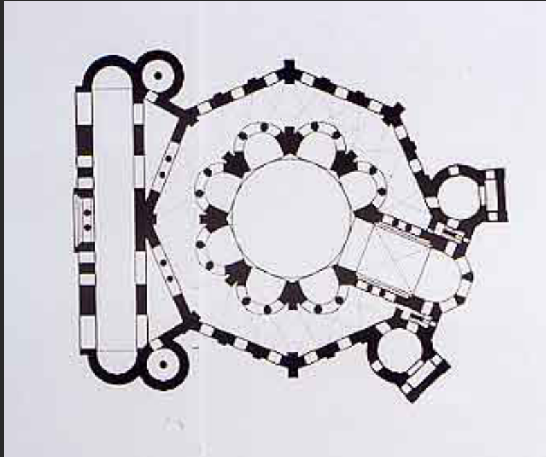
แปลนวัดซานไวทาลे เมืองราเวนนา โดมรูปแปดเหลี่ยม เส้นผ่าศูนย์กลาง 115 ฟุต ค.ศ. 526 - 547
