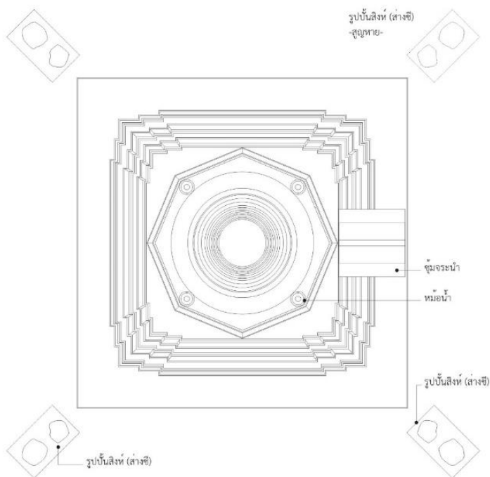
ภาพวาดลายเส้นแผนผังพระธาตุเจดีย์เมืองปอน
